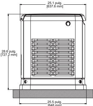
VISTA LATERAL IZQUIERDA
