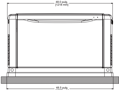
VISTA DELANTERA
